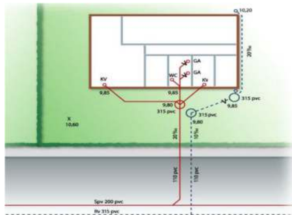
Principskitse over en typisk afløbsinstallation
